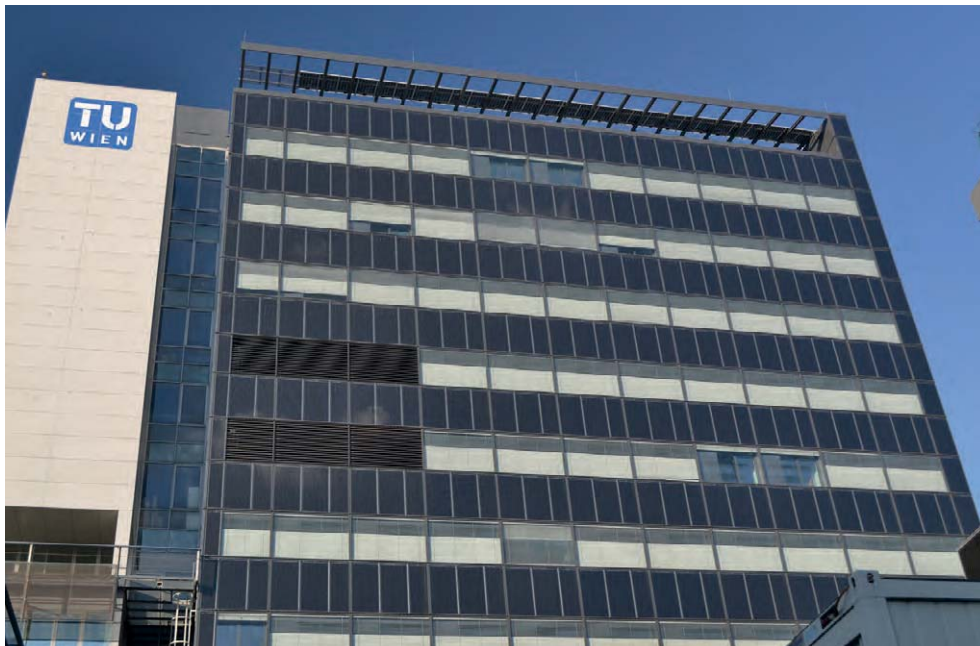
Die Fassade des Chemiehochhauses der TU Wien wurde schon ursprünglich in einer Pfosten-Riegel-Bauweise errichtet. Hier wurden bei der Sanierung die inaktiven Elemente durch Solarmodule ersetzt. (© Velka Botička)
