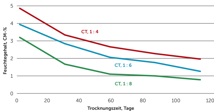
Abb. 1: Trocknung abhängig vom Zementgehalt
